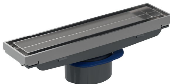
CleanLine personalizzabile, dettaglio dell'imbuto e della copertura
